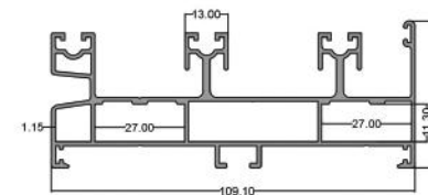
سیل عرق گیر سه ریل 3 Rails Takeout Steam Frame code: PNS6031 10.400 kg
