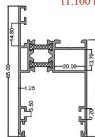
تا بیل ۸۵ Vent Profile 85 code: PMS6013 7.800 kg
