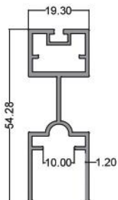
لنگه ریلی Sliding Vent code: MIS003 3.300 kg
