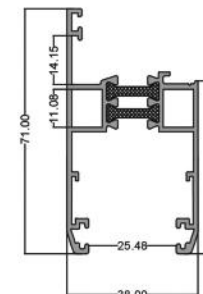
تابریل زهوار خور ۷۷ Vent On Rickety A Place 77 code: T392 5.700 kg
