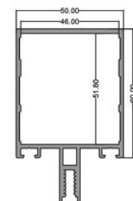
افقی ۶۰ Horizontal Profile 60 code: CWS60 8,400kg
