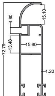
توری خور دسته دار Grid Frame With Handle code: PMS6019 4.100 Kg
