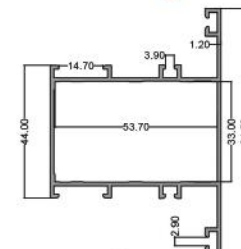
سپری ۶۵ Tirpetalous 65 code: N2 6.00kg
