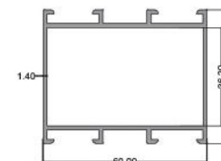
فریم ۶۰ Frame 60 code: PNP6001 6.100 kg
