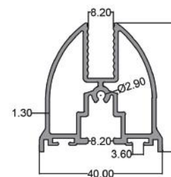
شیشه گیر جام بالکن Balcony Glass Holder code: BA02 5.200 kg
