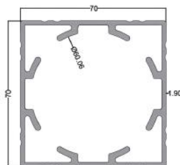
استارتر ۷۰ Starter 70 code: R124 11.400 kg
