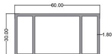
پروفیل ۶۰*۳۰ Profile 60*30 code: STR008 6.600kg
