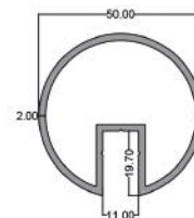
نگهدارنده شیشه پاسار Pasar Glass Holder code: PA02 6.200kg
