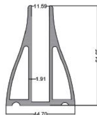
پاسار هلال Bend Over Pasar code: B11 9.600 kg
