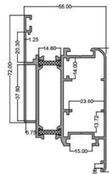
لنگه بزرگ پانچی Grand Vent code: PMH0013 11.300 kg
