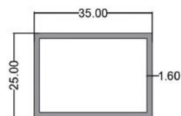
پروفیل ۲۵*۳۵ Profile 35*25 code: STR0011 3.600kg
