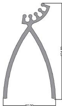
مقتاری چرخشی لوور Rotational Louver code: LO3 14.400 kg
