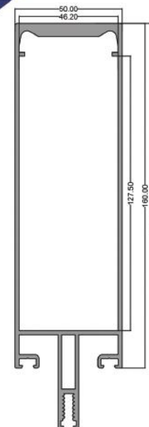
عمودی ۱۶۰ Vertical 160 code: CW353 19.500kg
