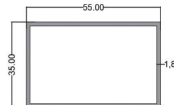
پروفیل ۵۵*۳۵ Profile 35*55 code: STR004T/1.8 5.150 kg
