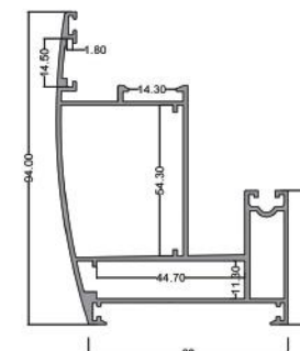
سیل منوریل Monorail Frame code: PMR0001 9.900 kg
