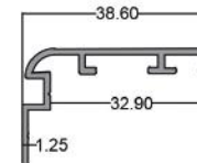
روکوب گرد Round Border code: PM00017 1.800 kg
