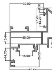
لنگه تخت ۴۴ Flat Vent 44 code: PNH4510 9.440 kg
