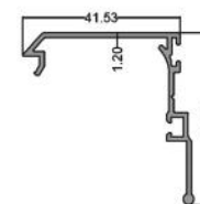
نیشی پشت لنگه ۷۷ Behind Vent Corner code: N394 2.500 kg
