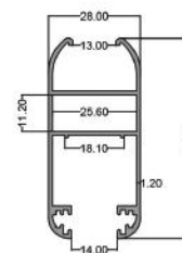
لنگه ریلی تک جداره Single- Walled Sliding Vent code: A10 4.300 kg
