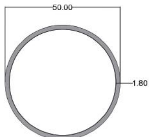
لوله ۵۰ Tube 50 code: R112-T1.80 4.500 kg
