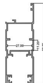
تابریل ۹۰ زهوار خور Vent On Rickety A Place 90 code: PNS6002 6.500 kg
