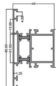
قید ریلی T - Profile code: PMS6021 7.00 kg
