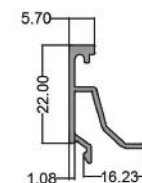
زهوار دو جداره Rickety ( Double Walled ) code: PNH0012 1.300 kg
