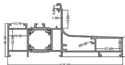
فریم بزرگ ۱۲۵ Grand Frame 125 code: PLH0007 12.100 kg
