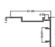
نبشی پشت لنگه ۹۰ Behind Vent Corner 90 code: PNS6010 2.300 kg
