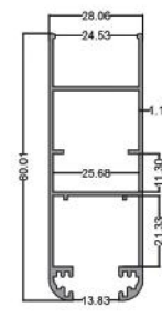
لنگه ریلی ۸۰ Sliding Vent 80 code: A5 5.00kg
