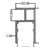
نگهدارنده شیشه Glass Holder code: PA05 3.00 kg
