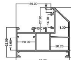
فریم تخت ۶۰ Flat Frame 60 code: PNH6010 10.405 kg
