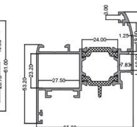
لنگه بازشو کوچک Small Opening Vent code: PLH0005 8.00 kg
