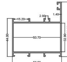
فریم ۶۵ Frame 65 code: N1 5.900kg
