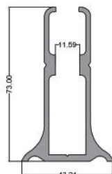
نرده پاسار Pasar Railing code: PA01 9.00 kg
