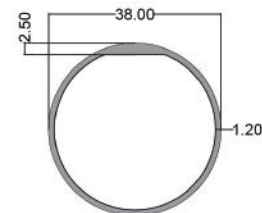
لوله ۳۸ Tube 38 code: R119 2.500kg
