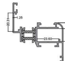
لنگه کوچک Small Vent code: PMH0011 6.600 kg
