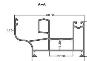
سیل توری خور تک تیغه Single Blade Grid Frame code: PNS6017 6.900 kg
