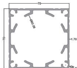
استارتر پیچ خور ۷۰ Starter 70 code: R.S124 12.00 kg
