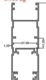
تابریل ۹۰ Vent Profile 90 code: PNS6024 7.00 kg
