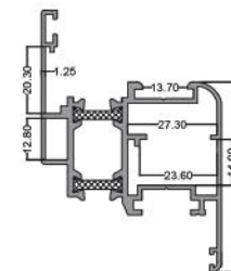
لنگه متوسط Average Vent code: PMH0012 8.400 kg
