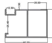
هندریل زهوار خور Hand Rail With Rickety code: B7 5.300kg
