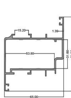
لنگه کوچک ۶۵ Small Vent 65 code: N12 7.200kg
