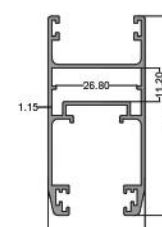
تابریل ۷۰ Vent Profile 70 code: PNS6013 5.200 kg
