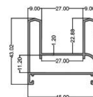
چهارچوب ریلی ۴۵ Sliding Rectangular 45 code: A9 4.500 kg
