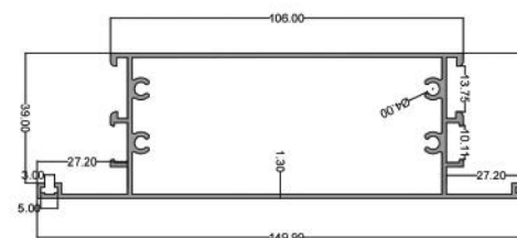
سپری ۱۵۰ Tripetalous 150 code: PNS6021 13.800 kg
