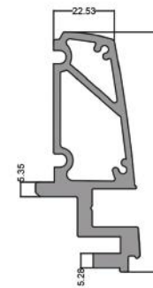
نرده پاسار پیچ خور Screw Paser Railing code: PA502 14.200kg
