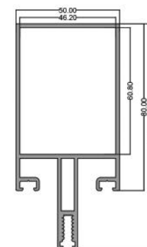
عمودی ۸۰ Vertical 80 code: CW80 11.700kg
