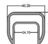
پروفیل شیشه گیر Stuck Glass Profile code: PA505 6.00kg
