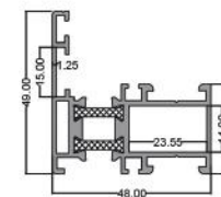
فریم کوچک ۴۸ Small Frame 48 code: PMH4811 6.600 kg
