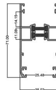
تابریل ۷۷ Vent Profile 77 code: N4.N4 9.160 kg
