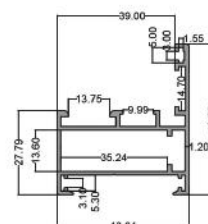
فریم تخت ۴۴ Flat Frame 44 code: PNH4511 6.720 kg
