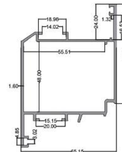
لنگه بزرگ Grand Vent code: LB418 8.800kg
