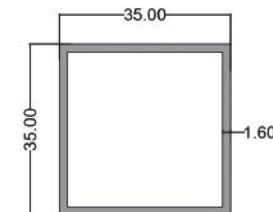
پروفیل ۳۵*۳۵ Profile 35*35 code: STR003 3.500kg
