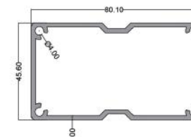
فیکسر عمودی Vertical Fixer code: CWS007 8.700kg
