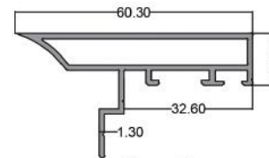
روکوب ۶۰ Border 50 code: RM00017 3.600 kg
