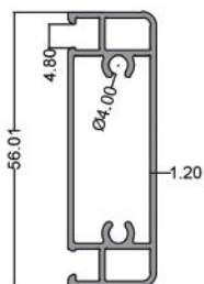
قید توری Grid T Profile code: PNS6026 4.00 Kg
