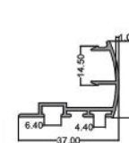
نیشی پشت لنگه Behind Vent Corner code: K336-3 1.800kg
