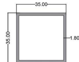
پروفیل ۳۵*۳۵ Profile 35*35 code: STR002 3.900kg
