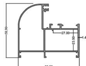
فریم ۷۰ Frame 70 code: A1 5.900 kg
