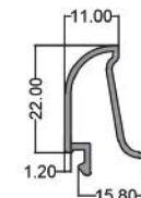
زهوار گرد دو جداره Round Rickety ( Double Walled ) code: PM00011 1.400 kg
