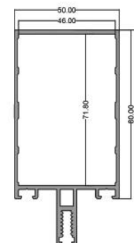
افقی ۸۰ Horizontal Profile 80 code: CWS80 9,300kg
