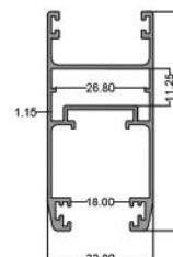
تابریل ۷۰ Sliding Vent code: N356 5.100 kg
