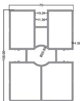
پایه چهار گوش ۱۰۰×۷۰ Grooved Rectangular Profile 70 X 100 code: B4 14.300 kg
