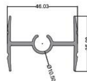
پروفیل پایه لوور Baic Louver Profile code: LO2 3.900 kg
