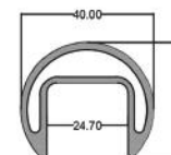
پروفیل شیشه گیر Stuck Glass Profile code: PA504 5.200kg
