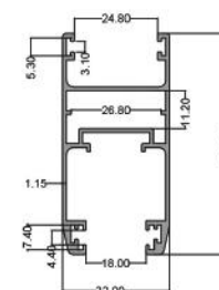
تابریل ۶۰ Vent Profile 60 code: PNS6013 5.100 kg
