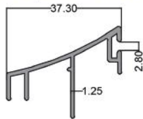
درپوش باران گیر Rain Cap code: PNS6019 2.200 kg
