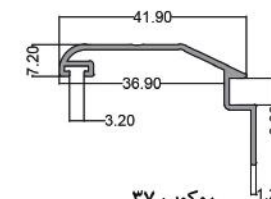
روکوب ۳۷ Border 37 code: RN00012 1.800 kg
