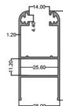
تایرل Sliding Vent(Vent Profile) code: K336-4 4.200kg
