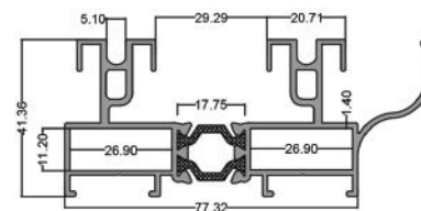
چهار چوب توری خور Grid Frame Rectangular code: F391 10.200 kg
