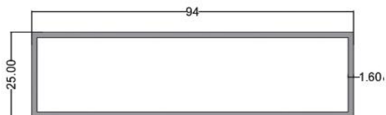
پروفیل ۹۴*۲۵ Profile 94*25 code: STR009 6.300kg
