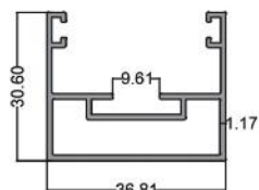
فریم Frame code: MIS004 3.200 kg
