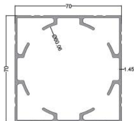
استارتر ۷۰ Starter 70 code: IQ8 9.00 kg
