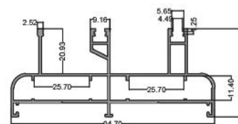
چهارچوب ریلی ۹۵ Sliding Rectangular 95 code: A3 7.800kg
