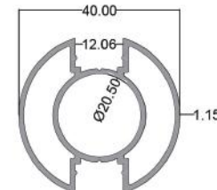
پایه دوطرفه ۴۰ Double Sided Base 40 code: R117 6.00 kg
