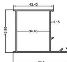
فریم سبک ۴۵ Light Frame 45 code: R1 3.800 kg
