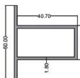
سپری Tripetalous code: STS0016 4.450 kg
