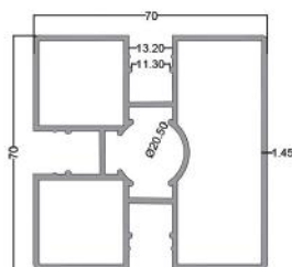
پایه چهار گوش شیاردار ۷۰×۷۰ Grooved Rectangular Profile 70 X 70 code: B3 10.500 kg
