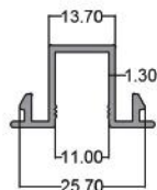
زهوار تبدیل Conversion Rickety code: PNH0010 2.400 kg
