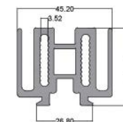
فیکس افقی Horizontal Fixer code: CWS008 11.500kg
