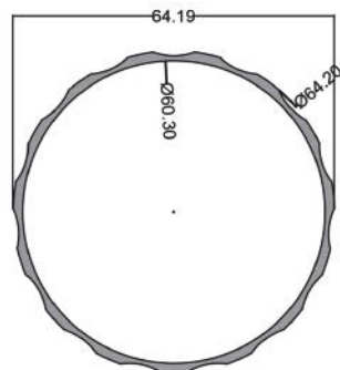
لوله ۶۳ Tube 63 code: IQ 2 5.00kg
