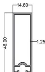
آدابتور جدید New Adapter code: PNS6026 2.700kg
