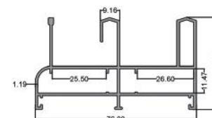
چهارچوب ریلی ۷۵ Sliding Rectangular 75 code: A4 6.600kg
