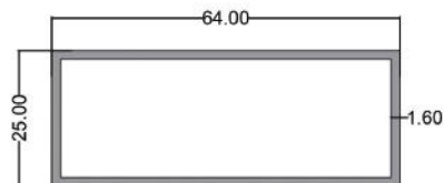
پروفیل ۶۴*۲۵ Profile 25*64 code: STR007 4.600kg
