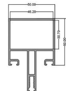
عمودی ۵۰ Vertical 50 code: CW50 9.800kg
