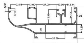
سیل عرق گیر Take Out Steam Frame code: PNS6018 8.300 kg
