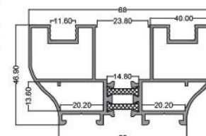
چهار چوب (سیل ساده) Grid Frame Rectangular (Frame Profile) code: PMS6011 10.00 kg
