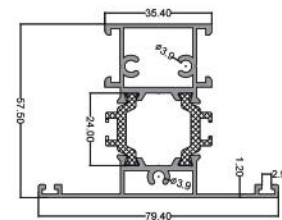
سپری ۸۰ Tripetalous 80 code: PLH0003 7.900 kg
