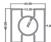
چهار گوشه دو طرفه ۴۰ Double Sided Rectangular 40 code: R126 5.400 kg
