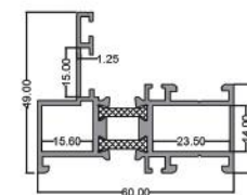
فریم تخت ۶۰ Flat Frame 60 code: PMH6012 7.200 kg
