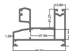
سیل تک تیغه Single Blade Frame code: PNS6006/1 6.00 kg
