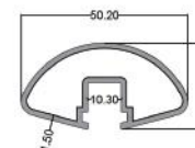
هندریل گرد شیشه خور Round Hand Rail On Glass A Place code: B9 3.600 kg
