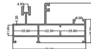
چهارچوب ۸۰ Sliding Rectangular 80 code: K336-8 6.500kg
