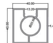
چهار گوشه یک طرفه ۴۰ Single Sided Rectangular 40 code: R120 5.400 kg
