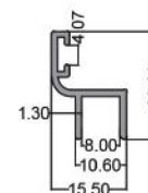
شیشه گیر لنگه Balcony Glass Frame code: BA05 1.100 kg
