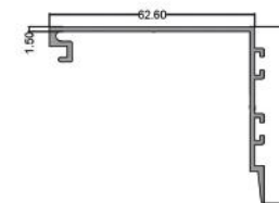
نبشی پشت لنگه Behinde Vent Corner code: PLS0005 3.700 kg
