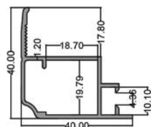
پروفیل درب یخچالی شیاردار Profile code: Y424 0kg
