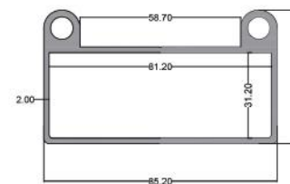
دیوار کوب Conection To Wall Bracket code: R5 11.100 kg
