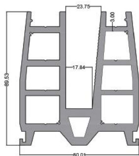
نرده پاسار بزرگ Grand Pasar Railing code: PA03 38.300 kg
