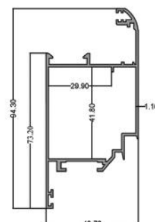
لنگه بزرگ Grand Vent code: A8 5.600 kg
