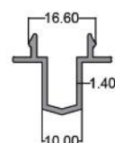
آدابتور قدیم Old Adapter code: PNS6023 1.400kg
