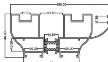
چهار چوب توری خور (سیل توری خور) Grid Frame code: PMS6012 11.100 kg
