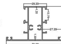
سپری تخت ۷۰ Flat Tripetalous 70 code: PNS6027 8.210 kg
