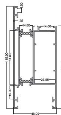
لنگه فرجه خور Vent on Brush A Place code: PMH6014 12.00 kg
