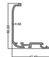
نبشی پشت لنگه ۱۰ Behind Vent Coner 10 code: PMS6015 3.00 kg
