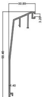
دربوش پاسار بزرگ Grand Pasar Cap code: PA04 3.500 kg
