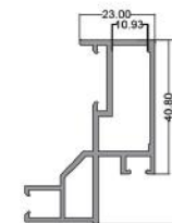
لنگه Vent code: CWS001 5.00kg
