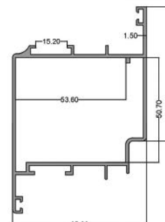
لنگه بزرگ ۶۵ Grand Vent 65 code: N3 8.00kg
