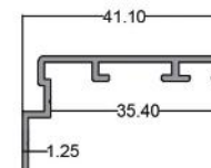
روکوب تخت Flat Border code: PM00016 1.800 kg
