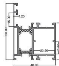
فریم بزرگ ۴۸ Grand Frame 48 code: PMH4812 7.900 kg
