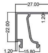
زهوار تخت تک جداره Flat Rickety ( Single Walled ) code: PM00015 1.900 kg
