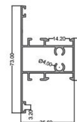
سپری ۷۰ Tripetalous 70 code: PNH4813 5.00 kg
