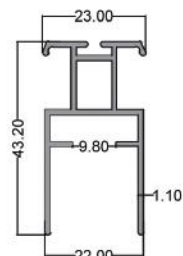
لنگه ریلی Sliding Vent code: N15 2.600 kg
