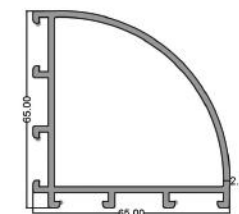
فریم گوشه گرد Round Corner Frame code: PNP6006 8.600 kg
