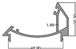
کوپلینگ Coupling code: PN00018 4.300 kg
