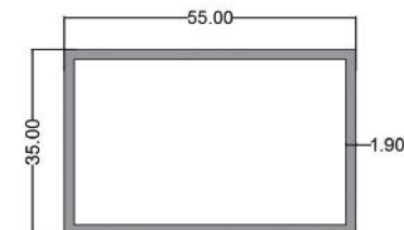
پروفیل ۵۵*۳۵ Profile 35*55 code: STR005 5.350kg
