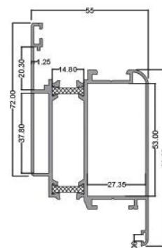
لنگه بزرگ (هیدرولیک) Grand Vent code: PMH0015 11.100 kg
