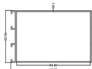
فریم ۱۰۰ Frame 100 code: PNP6004 9.00 kg
