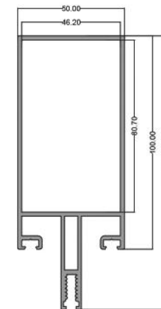
عمودی ۱۰۰ Vertical 100 code: CW100 12.900kg
