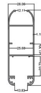
لنگه ریلی تک جداره Single-Walled Sliding Vent code: A6 5.200 kg
