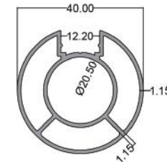
پایه یک طرفه ۴۰ Single Sided Base 40 code: R113 4.00 kg
