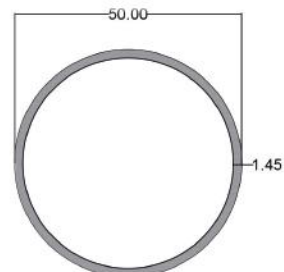
لوله ۵۰ Tube 50 code: R112-T1.45 3.700 kg
