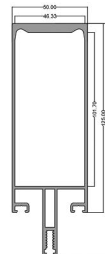
عمودی ۱۲۵ Vertical 125 code: CW120 17.200kg
