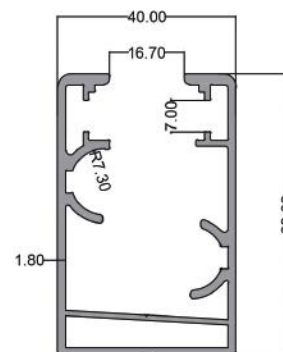
ریل جام بالکن Balcony Rail code: BA01 8.100 kg
