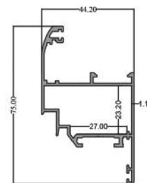
لنگه کوچک Small Vent code: A2 5.00 kg
