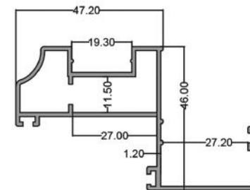
لنگه ثابت Fixed Vent code: FLS002 5.00 kg
