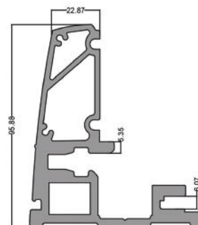
نرده پاسار مهره خور Nut Paser Railing code: PA501 24.300kg
