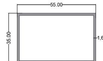
پروفیل ۵۵*۳۵ Profile 35*55 code: STR004T/1.6 4.750 kg
