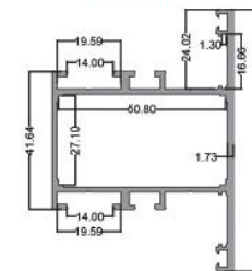
سپری Tripetalous code: S416 7.600kg
