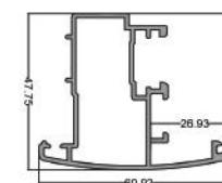
دولنگه تخت Flat Double Vent code: PNS6028 7.450 kg
