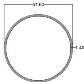
لوله ۵۱ Tube 51 code: R118-T1.40 5.900kg
