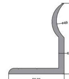
نگهدارنده لوله ۵۰ Tube Holder 50 code: R128 11.800 kg
