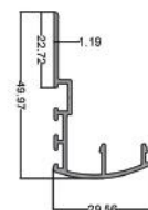
نبشی پشت لنگه هلال Bend Behind Vent Corner code: A7 2.300 kg
