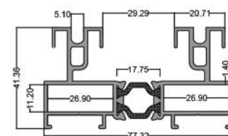
چهار چوب Rectangular code: F390 9.00 kg
