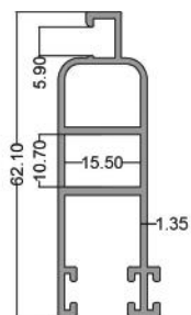
توری خور قدیم Old Grid Frame code: PNS6022 4.300 Kg
