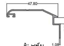
روکوب ۵۰ Border 50 code: RN00013 1.700 kg
