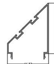
زاویه ۹۰ ترمال بریک Angle Profile 90 (Thermal Break) code: ZT90 4.00 kg
