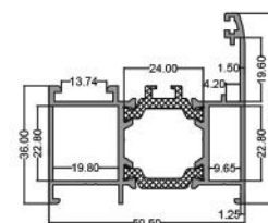
فریم بزرگ ۶۰ Grand Frame 60 code: PLH0001 7.00 kg
