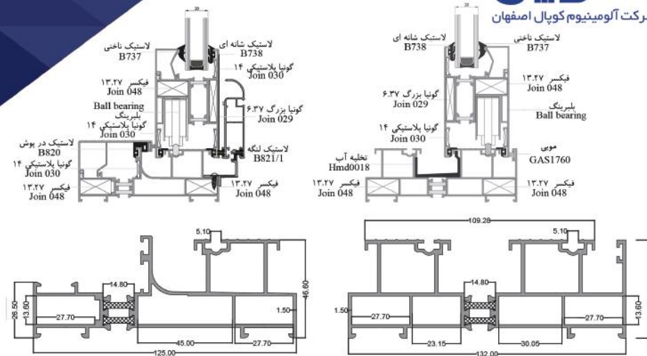
سیل تک ریل منوریل Single Rail Frame (Monorail) code: PLS0002 13.200 kg
