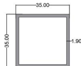
پروفیل ۳۵*۳۵ Profile 35*35 code: STR001 4.100 kg
