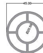
نگهدارنده استارتر Starter Holder code: R127 7.900 kg
