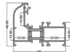
فریم ۶۰ گرد Round Frame 60 code: PMH6011 7.800 kg
