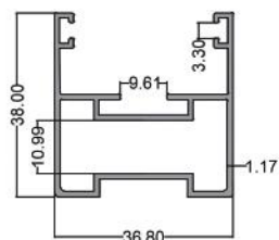
فریم فیکسر خور Frame On Fixer A place code: MIS005 3.500 kg
