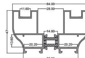
چهار چوب (سیل هلال) Bend Over Frame code: PMS6020 9.900 kg
