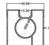
چهار گوشه یک طرفه تک جانبی ۴۰ Lateral 1Base Single Sided Rectangular 40 code: B6 4.600 kg
