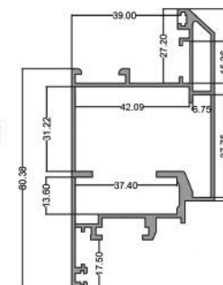
لنگه تخت ۶۰ Flat Vent 60 code: PNS6029 12.190 kg
