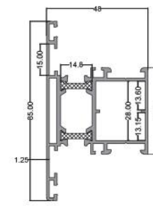
سپری ۸۵ Tripetalous 85 code: PMH6013 8.600 kg
