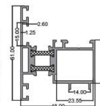
دولنگه Double Vent code: PMH4913 6.900 kg
