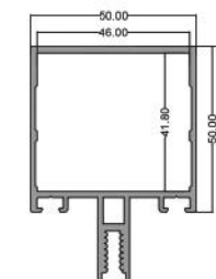
افقی ۵۰ Horizontal Profile 50 code: CWS50 7,900kg
