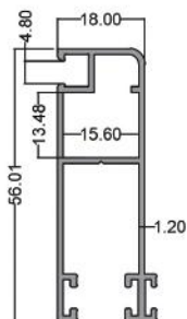
توری خور ساده Simple Grid Frame code: PMS6025 3.600 Kg
