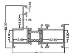
فریم ۶۰ تخت Flat Frame 60 code: PMH6012 7.200 kg
