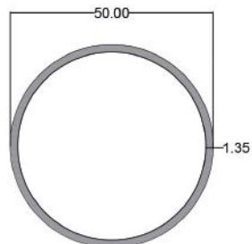
لوله ۵۰ Tube 50 code: R112-T1.35 3.400 kg
