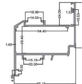
لنگه کوچک Small Vent code: LK419 8.00kg
