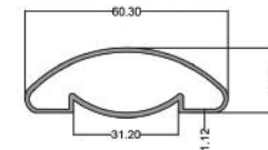
هندریل گرد Round Hand Rail code: IQ3 3.100kg
