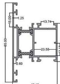
سپری ۸۵ Tripetalous 85 code: PMH6013 8.600 kg
