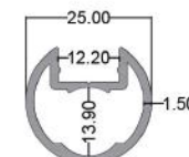
لوله ۲۵ Tube 25 code: R115 2.200kg
