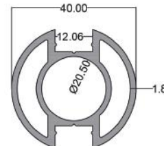
پایه دوطرفه ۴۰ Double Sided Base 40 code: R116 6.100 kg
