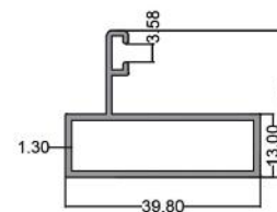
فریم جام بالکن Balcony Frame code: BA03 2.700 kg
