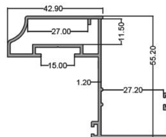
لنگه لولایی Hinged Vent code: FLS001 5.00 kg
