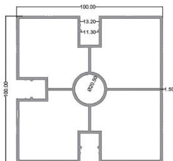
پایه چهار گوش ۱۰۰×۱۰۰ Rectangular Profile 100 X 100 code: B5 16.400 kg
