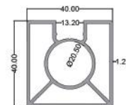
چهار گوشه یک طرفه ۴۰ Single Sided Rectangular 40 code: R122 5.400 kg
