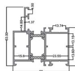
فریم ۶۰ تخت بلند Long Flat Frame 60 code: PMH6015 8.700 kg
