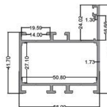
فریم ۵۵ Frame 55 code: F417 6.900kg
