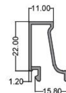
زهوار تخت دو جداره Flat Rickety ( Double Walled ) code: PM00012 1.500 kg
