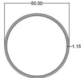
لوله ۵۰ Tube 50 code: R112-T1.15 3.00 kg
